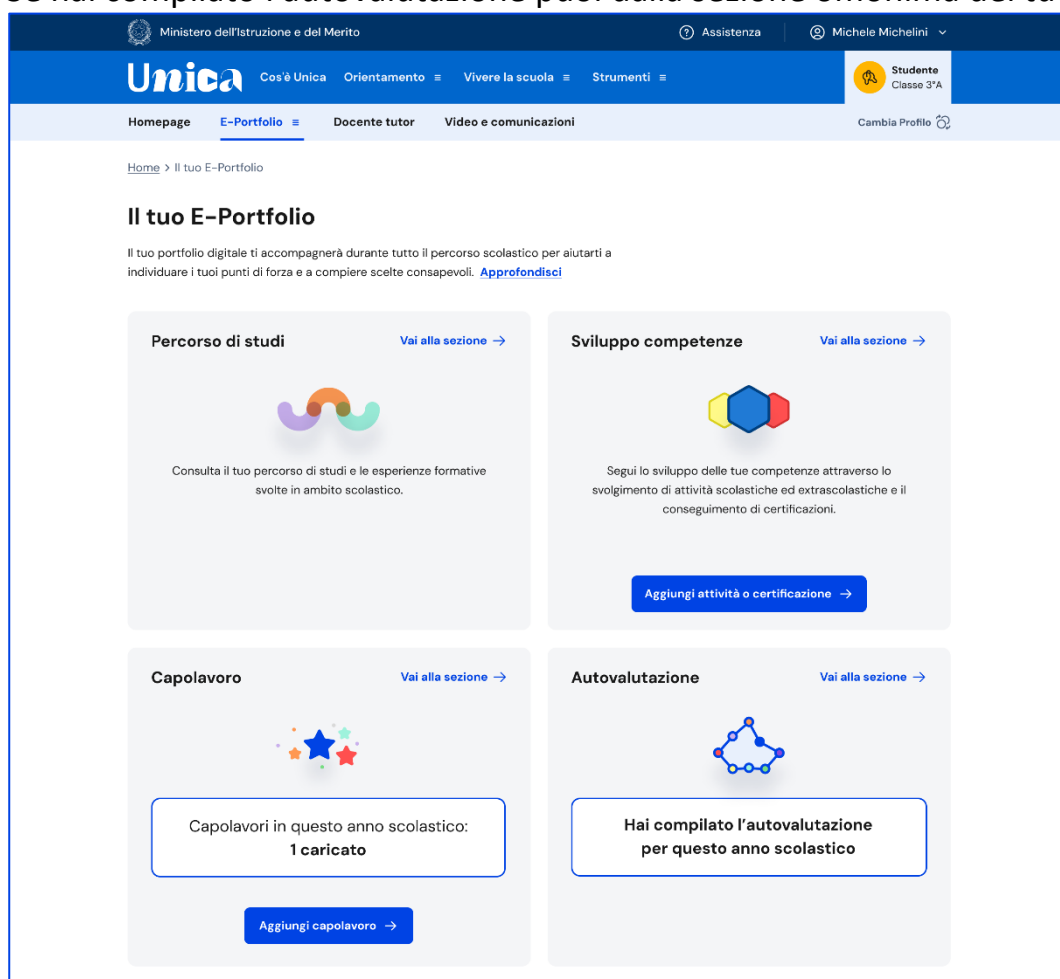
FIGURA 51 –SCHERMATA E-PORTFOLIO/AUTOVALUTAZIONE
